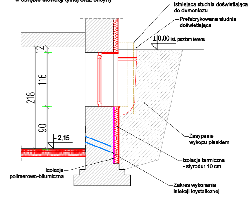
Przekrój przez studzienkę doświetlającą w obrębie elewacji tylnej oraz oficyny
