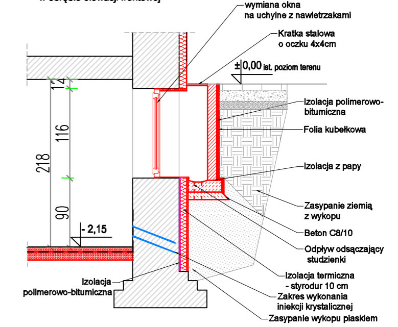
Przekrój przez studzienkę doświetlającą w obrębie elewacji frontowej
